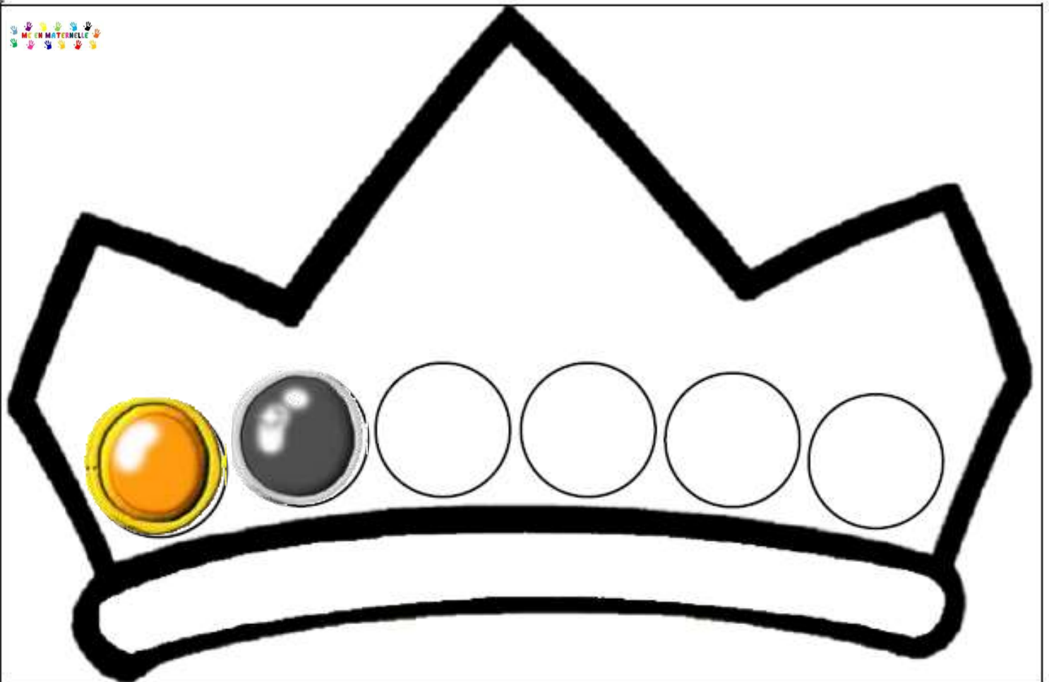
Algorithmes des couronnes
